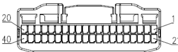
Рисунок 6 - Вид (со стороны изделия) на контакты соединителя питания и интерфейсов Блока УВЭОС-07
